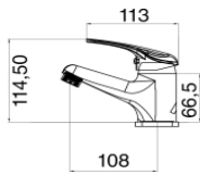
Mix Lavabo con basetta e flessibili e scarico automatico Cartuccia D. 40
