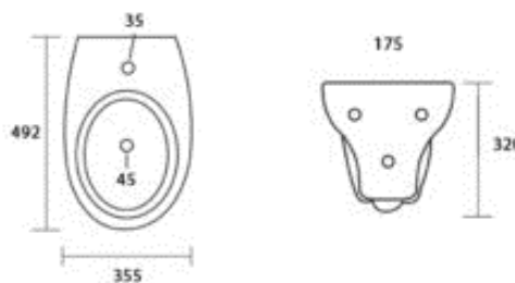
BIDET NEPI SOSPEO 360X500X340 IN CERAMICA BIANCO LUCIDO 1756.30
