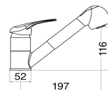
Mix Lav. Mon. Doc /Estr. Debora Cartuccia 40 MLMEDE00
