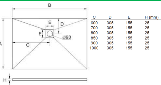
Piatto Doccia Stone Resina Effetto Ardesia Cod. 2100
