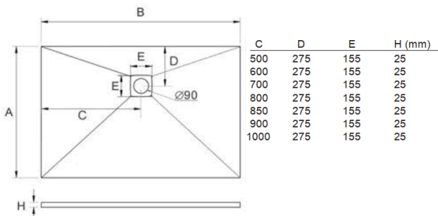
Piatto Doccia Stone Resina Effetto Ardesia Cod. 2100
