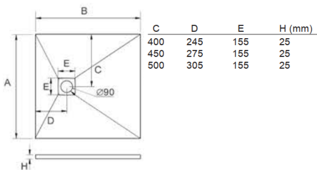
Piatto Doccia Stone Resina Effetto Ardesia Cod. 2090
