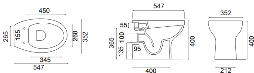
Cod. 1757.00 Vaso Oggi P 360x550x395 mm in Ceramica
