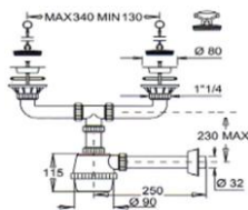
Sifone 2 Vie 11/4" Con Pilette S2V11\4C
