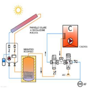
S142 Doppia Valvola Ritegno 93S142AE05
