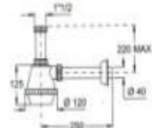
Sifone Moplen 1 V. 11/2" Magnum Tutto 11/2" S1V11\2M
