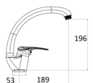
Mix Lavello Mon. Later. Debora Canna Alta Pesante Cromo MLMLDE00
