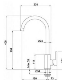
Mix Elleci C01 Avena 51 MGKC0151
