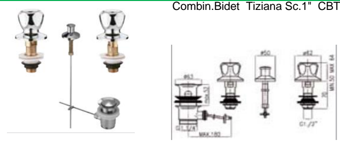
Combin.Bidet Tiziana Sc.1" CBT
