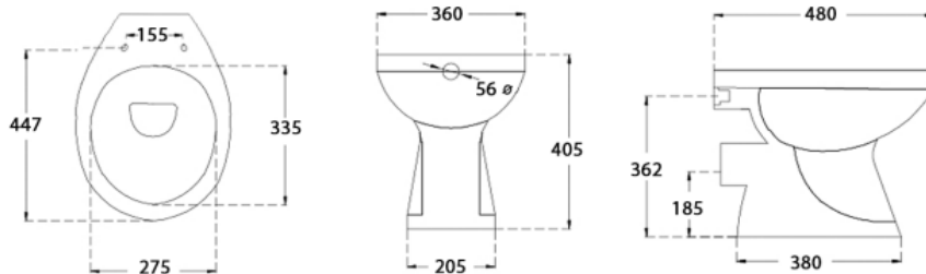
VASO CIVITA P.360X480X405 IN CERAMI CA BIANCO
