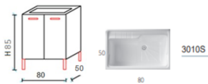
Lavatoio 80X50 Basic Con Piedini E Strofinatoio In Legno BB85
