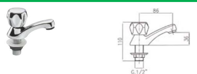
Rubinetto Collo Cigno 1/2" Tiz. RCT
