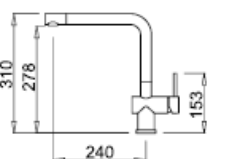
Miscelatore Cucina Con Doccetta Estraibile Rubinetto Monocomando Colore Cromo Nero MGKC0240
