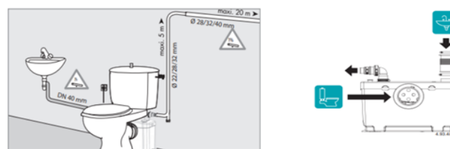
VASO+ATTACCO LAVABO
