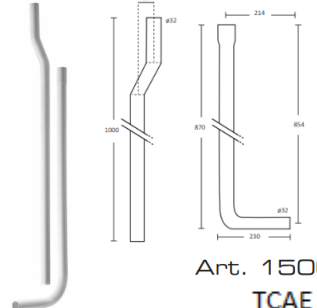
Tubo Cassetta Alta Esterno TCAE
