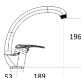
Mix Lavello Mon. Later. Debora Canna Alta Pesante Cromo MLMLDE00
