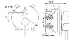
Miscelatore incasso 3 vie composto da: deviatore meccanico con easy box placca esterna
