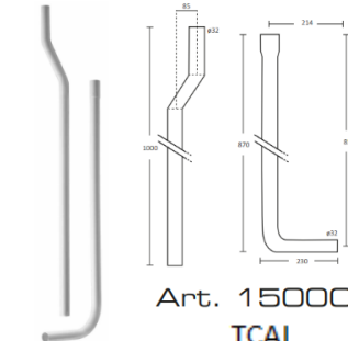
Tubo Cassetta Alta Incasso TCAI
