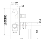
Miscelatore Doccia Incasso Con Deviatore Serie Nx Piastra Quadra
