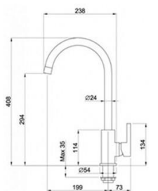
Mix Elleci C01 Nero 40 MGKC0140
