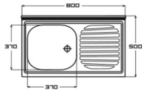
Lavello 80X50 1 Vasca Piu Gocciolatoio Destra - Serie Pisa Prelucido PI801RPC
