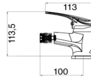
Mix Bidet con basetta e flessibili e scarico automatico Cartuccia D. 40
