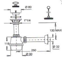
Sifone 1 Via Moplen Da 11/4" Con Piletta S1V11\4C
