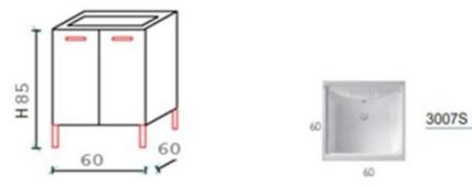
Lavatoio 60X60 Basic Con Piedini E Strofinatoio In Legno BB66
