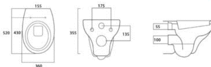
VASO NEPI SOSPEO P.360X510X365 IN CERAMICA BIANCO LUCIDO 1756.20
