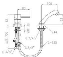
Monocomando parrucchiere "minimalista" con cartuccia Ø 35 mm flessibili di alimentazione in acciaio inox 70 cm. Flessibile in PVC grigio metallizzato 125 cm.
