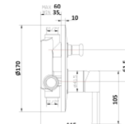
Miscelatore Doccia Incasso Con Deviatore Serie Mm MXDDMCMM3CR
