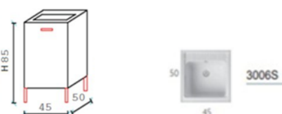
Lavatoio 45X50 Basic Con Piedini E Strofinatoio In Legno BB54
