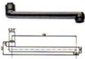
Bocca Erogazione a biscotto pesante
