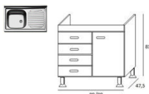
Kit Sottolavello 80X50 Teck Con Cassetti Sx Lavello Inox 80X50 1 Vasche Piu' G. Sx Bt5Ls+Pi801Lpc CL80CTLS
