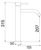
Lavabo Alto Serie Mm MXLHMCMMCCR
