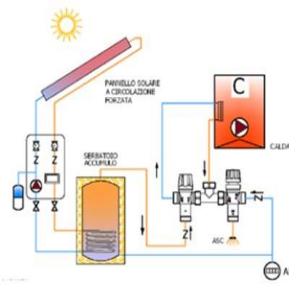
Kit Solare Miscelatore 1/2" KSCT12
