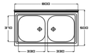
Lavello Appoggio 80X50 Cm 2 Vasche - Serie Pisa Prelucido PI802PC
