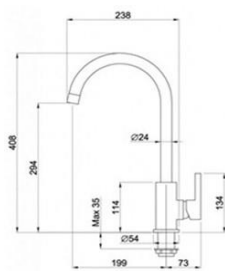
Mix Elleci C01 Chrome MIKC01CR
