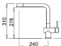
Miscelatore Cucina Con Doccetta Estraibile Rubinetto Monocomando Materiale Granitek Colore 51 Avena MGKC0251
