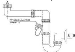
Sifone Lavello Autopulente A 1 Via 11/2" S/Piletta S1V11\2
