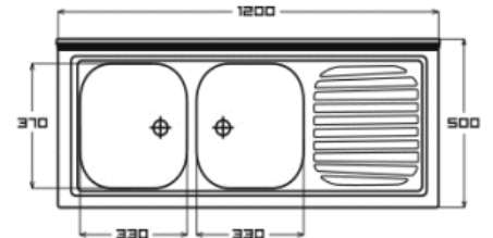
Lavello Appoggio 120X50cm Destra Serie Pisa Prelucido PI120RPC
