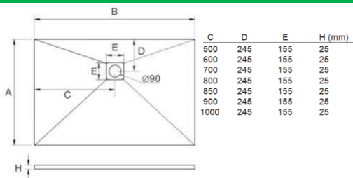
Piatto Doccia Stone Resina Effetto Ardesia Cod. 2100
