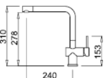
Miscelatore Cucina Con Doccetta Estraibile Rubinetto Monocomando Colore Cromo MIKC02CR
