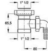
Attacco Lavatrice 11/2" Filettato Mf AL11\2F
